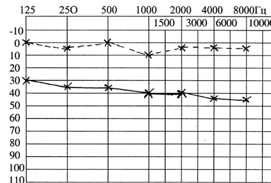
Аудиограмма №3
